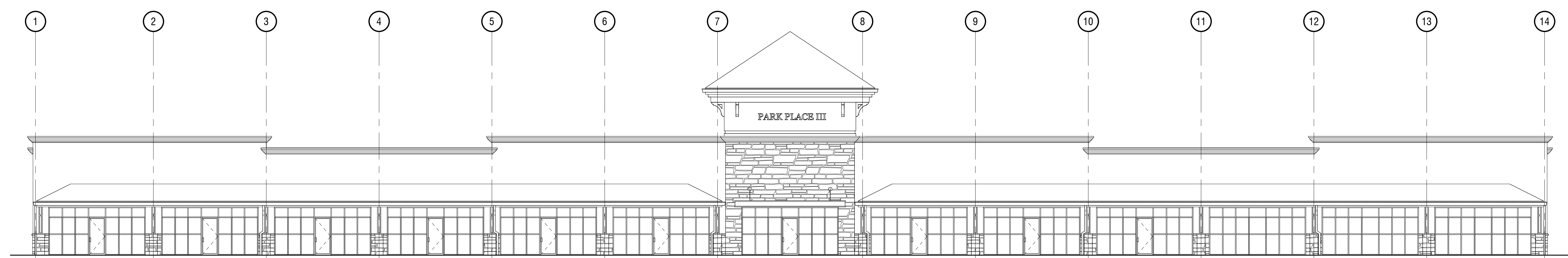
MAIN ELEVATION SCALE: 1" = 10'-0"
